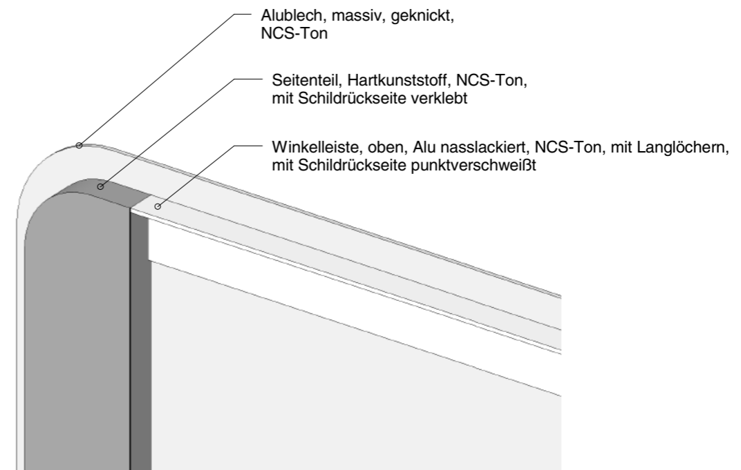
Aluplatte geknickt, Konstruktionsdetail
