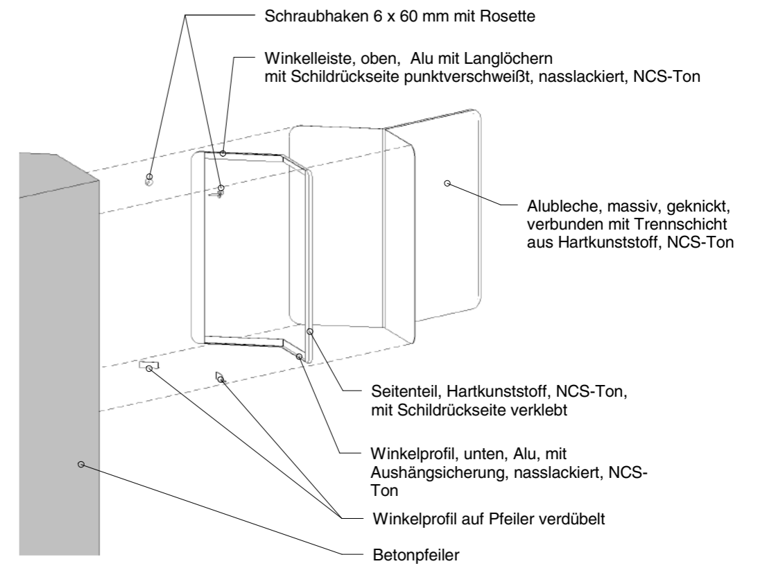
Aluplatte geknickt, Montagedetails
